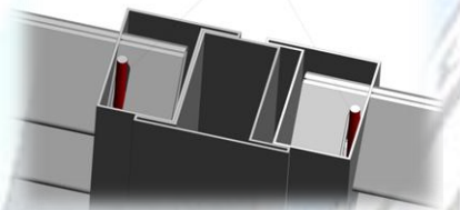
Particolare dei tondi in acciaio inox aisi 304 antistrappamento delle alette
