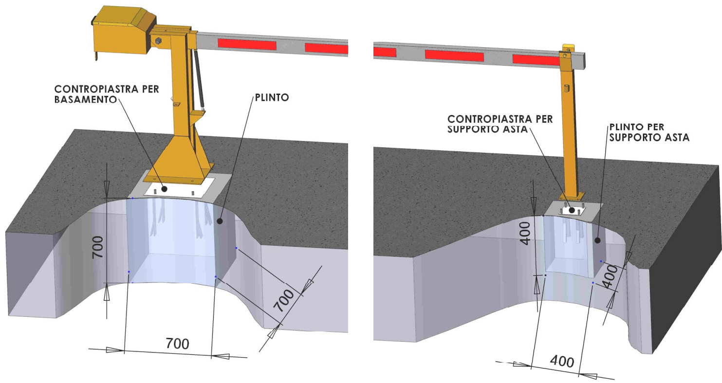
Barriere serie BM dimensionamento plinti
